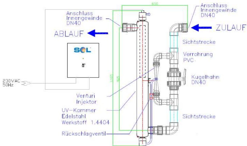
MAVOX – DUPLEX OZON–UV/SYSTEM(RS) TYPE 3 und 4 VENTURI VOR UV–ANLAGE
